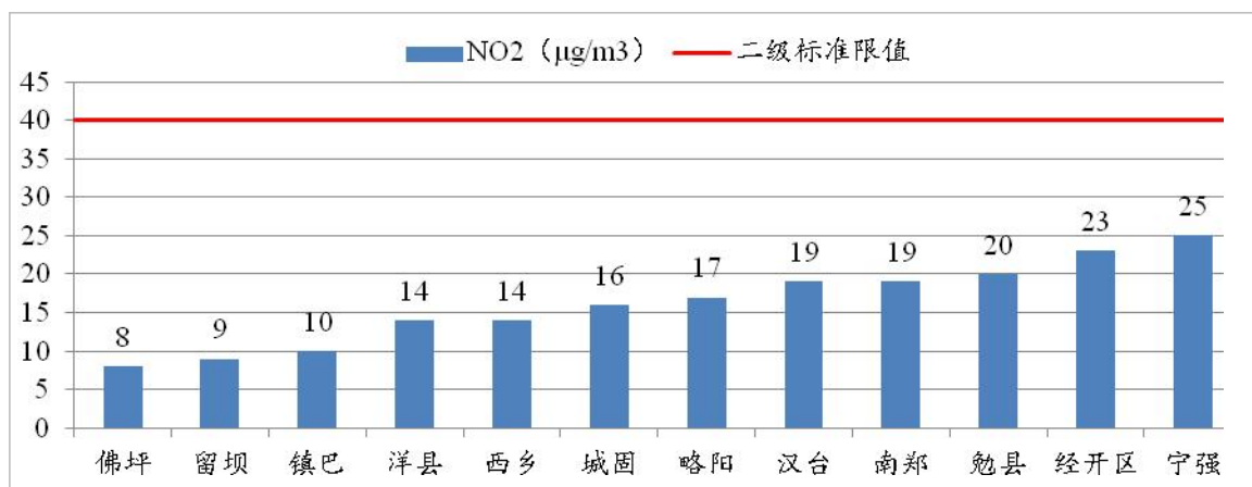
图 18 2022 年 1~12 月各县区 NO 2 浓度及达标情况
