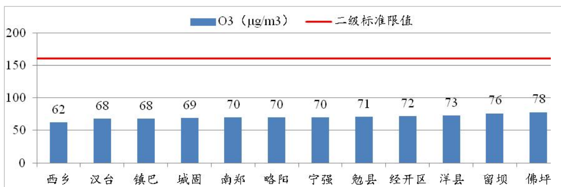
图10 2022年12月各县区O 3 浓度及达标情况
