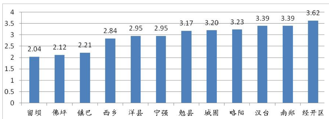
图 13 2022年1~12月县区环境空气质量综合指数
