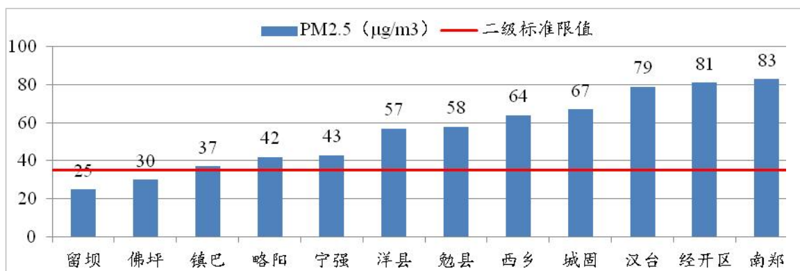
图6 2022年12月各县区PM 2.5 浓度及达标情况
