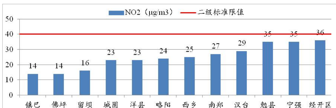
图8 2022年12月各县区NO 2 浓度及达标情况
