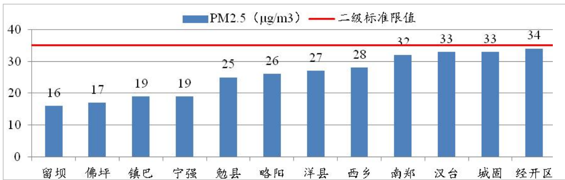
图 16 2022 年 1~12 月各县区 pM 2.5 浓度及达标情况
