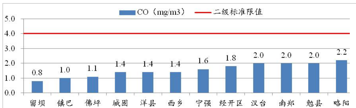
图9 2022年12月各县区CO浓度及达标情况
