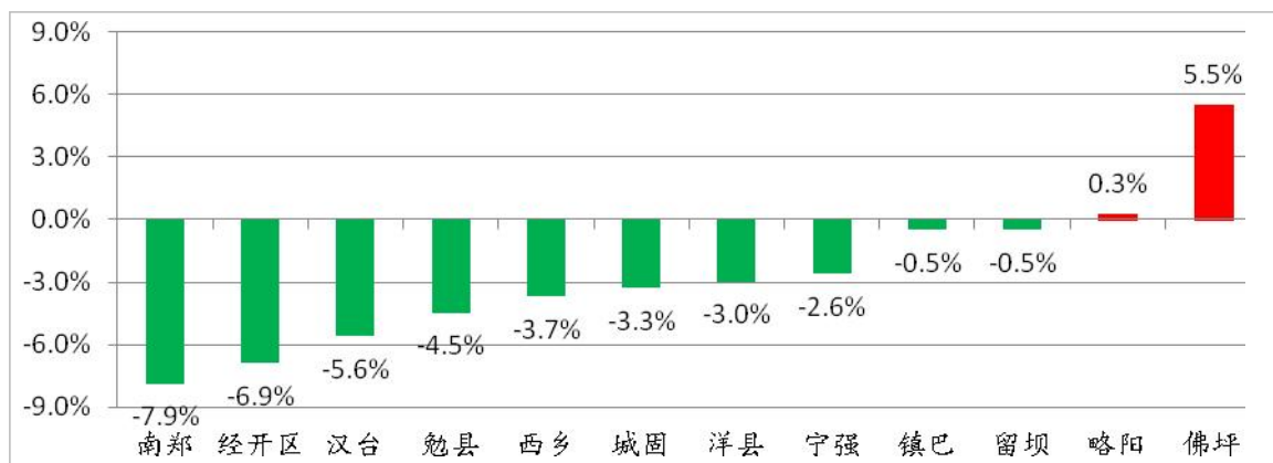
图 14 2022年1~12月县区环境空气质量综合指数同比变化情况
