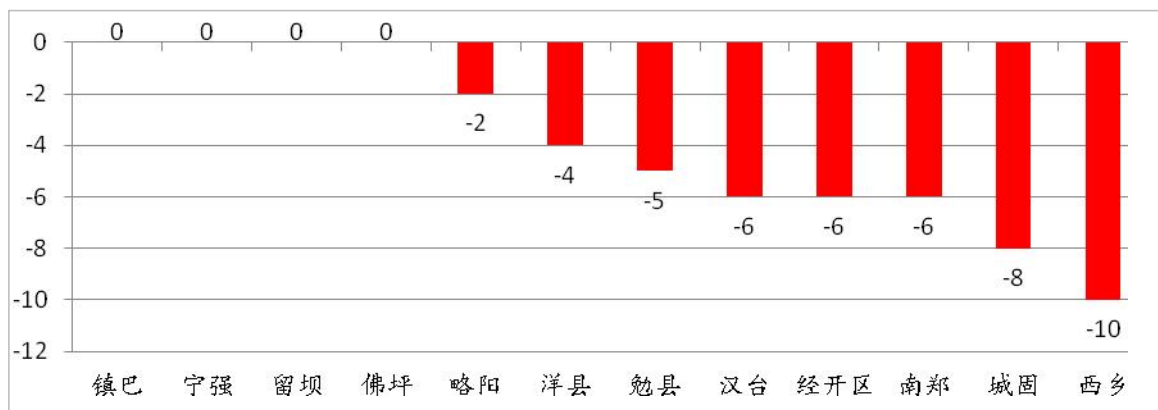
图2 2022年12月各县区环境空气质量优良天数同比变化情况 (单位: 天)
