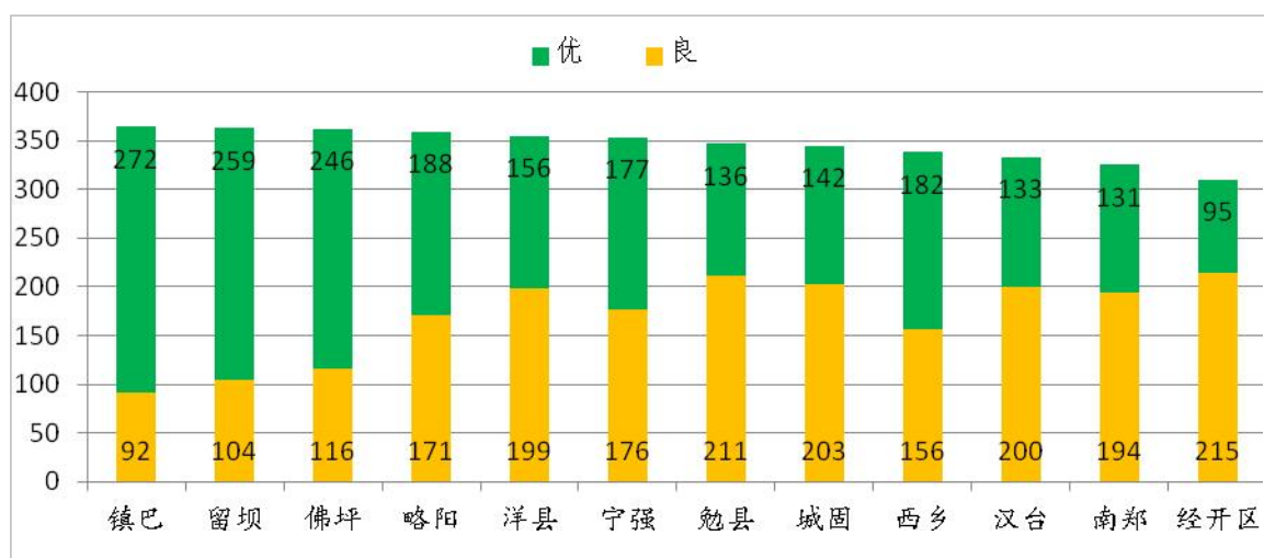
图 11 2022 年 1~12 月县区环境空气质量优良天数（单位：天）
