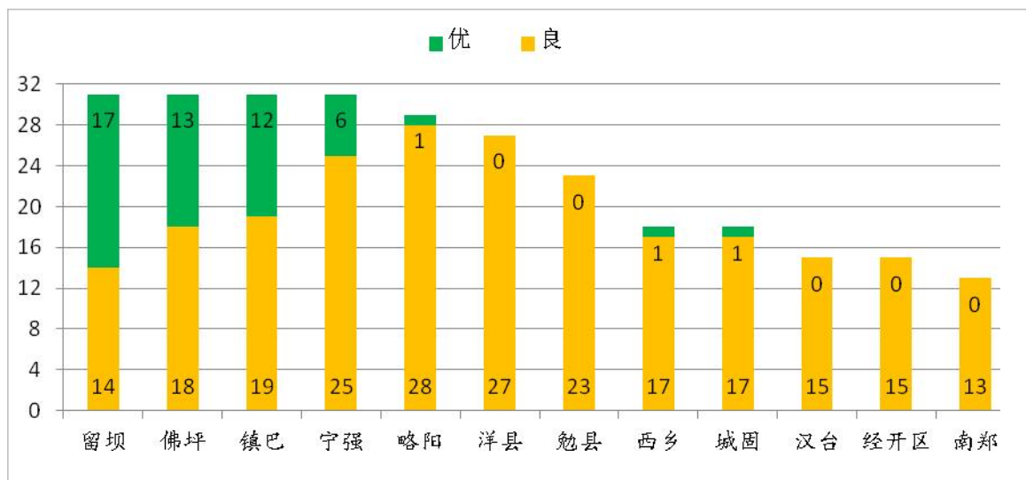
图1 2022年12月各县区环境空气质量优良天数图 (单位: 天)
