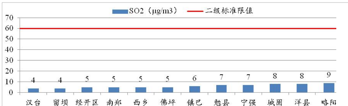
图 17 2022 年 1~12 月各县区 SO 2 浓度及达标情况
