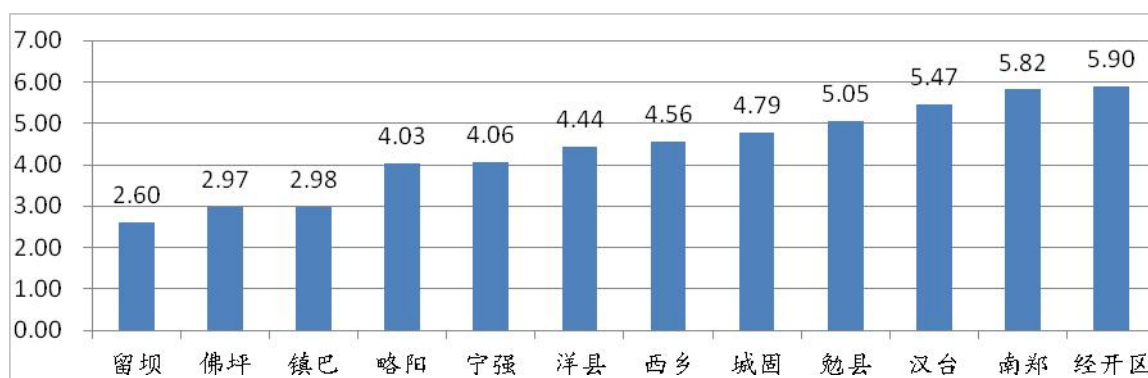
图3 2022年12月各县区环境空气质量综合指数
