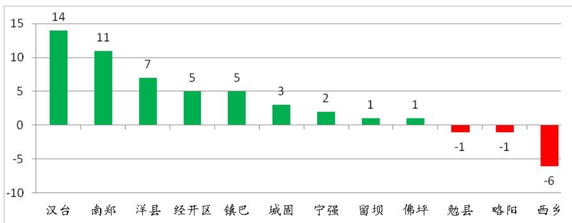
图 12 2022 年 1~12 月县区环境空气质量优良天数同比变化情况 (单位: 天)
