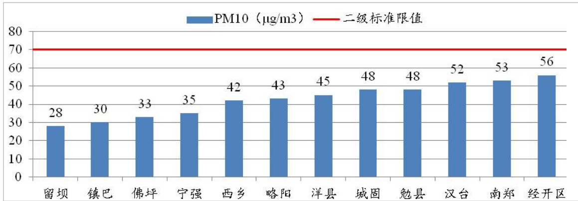
图 15 2022 年 1~12 月各县区 pM 10 浓度及达标情况
