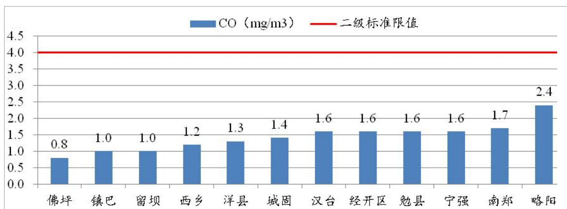
图 19 2022 年 1~12 月各县区 CO 浓度及达标情况
