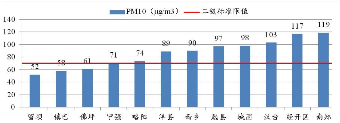
图5 2022年12月各县区 pM 10 浓度及达标情况
