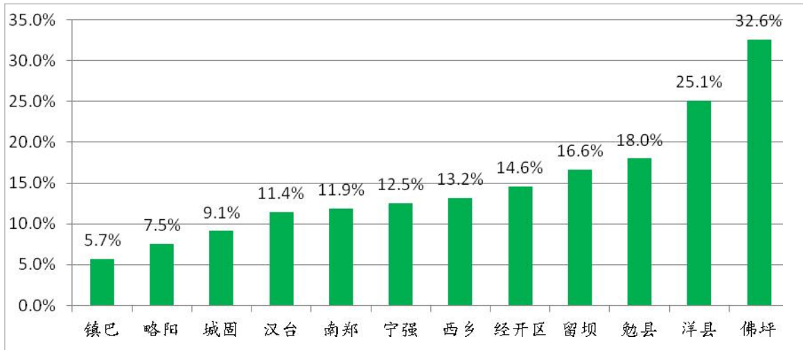
图4 2022年12月各县区环境空气质量综合指数同比变化情况
