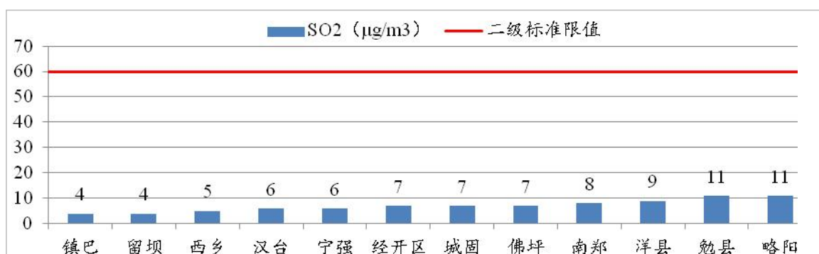
图7 2022年12月各县区SO 2 浓度及达标情况
