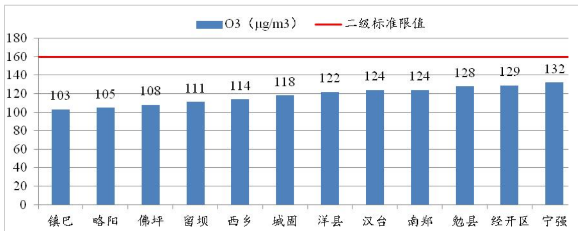
图 20 2022 年 1~12 月各县区 O 3 浓度及达标情况
